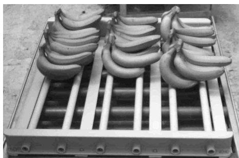
Figure 2. Prototype de plateau tubulaire sans fond : les fruits sont supportés par des barreaux espacés. Il ne peut plus y avoir d'eau résiduelle. Les rampes d'aspersion peuvent alors être disposées au-dessus et au-dessous du tray (photo J. Joas).
